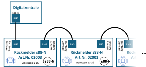
Abbildung 1: Anschluss an eine Digitalzentrale
