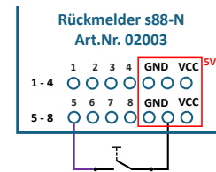
Abbildung 6: Anschluss eines Tasters/Reedkontaktes
