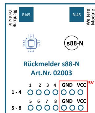
Abbildung 3: Übersicht über alle Anschlüsse des Rückmeldemoduls
