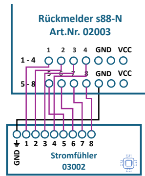
Abbildung 4: Anschluss eines Stromfühlers (Art.Nr. 03002)
