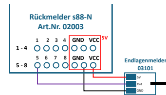
Abbildung 5: Anschluss eines Endlagenmelders (Art.Nr. 03101)
