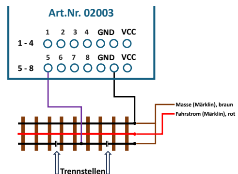
Abbildung 7: Anschluss eines Märklin Kontaktgleises
